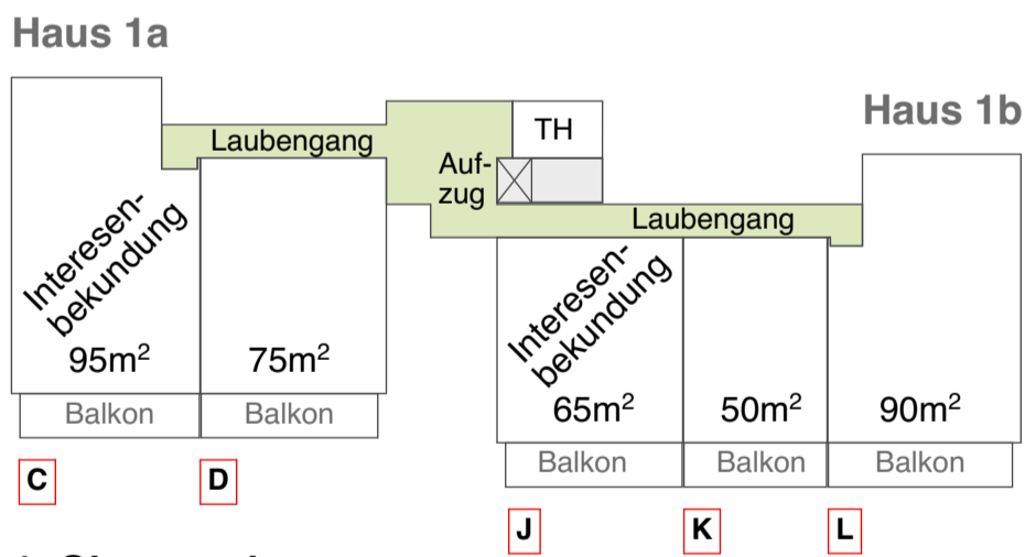
1. Obergeschoss
