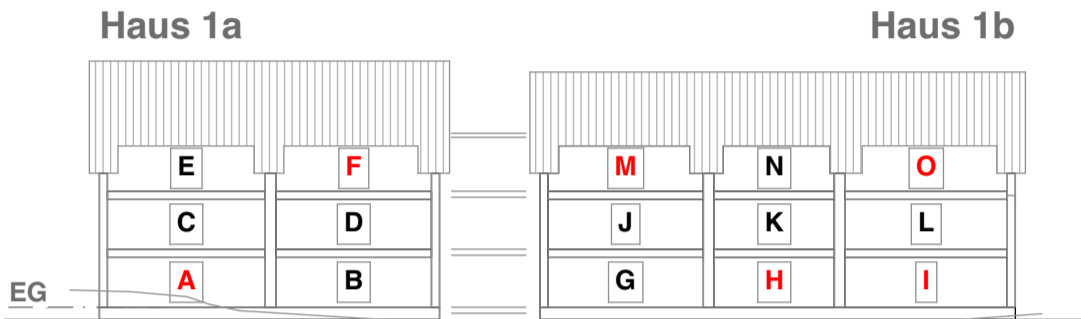
Ansicht Süd
